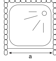
DUŞ TEKNESİ ÖN CEPHE ÖLÇÜLENDİRME
