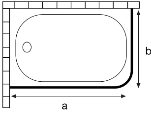
OTURMALI KÜVET 105'lik İKİ KENAR ÖLÇÜLENDİRME
