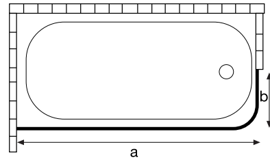
KÜVET ÜSTÜ ÖN CEPHE KENAR ÖLÇÜLENDİRME
